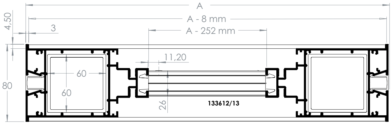
139738 Boormal T-verbinder [133612/13] Bohrschablone T-Verbinder Drilling template T-connector
