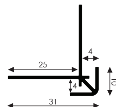
134226 Buitenhoekprofiel 4/4100 vom-1 (+T) External corner 4/4100 anod (+T) Außeneckprofil 4/4100 elox (+T)
